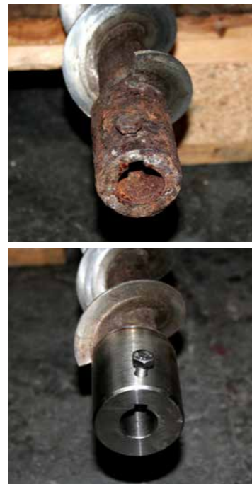
Kupplungsnahe (vorher-nachher)
