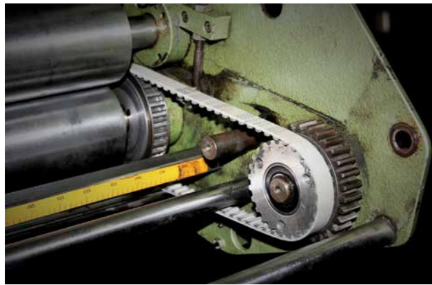
Zahnriemen-Antrieb gerichtet
